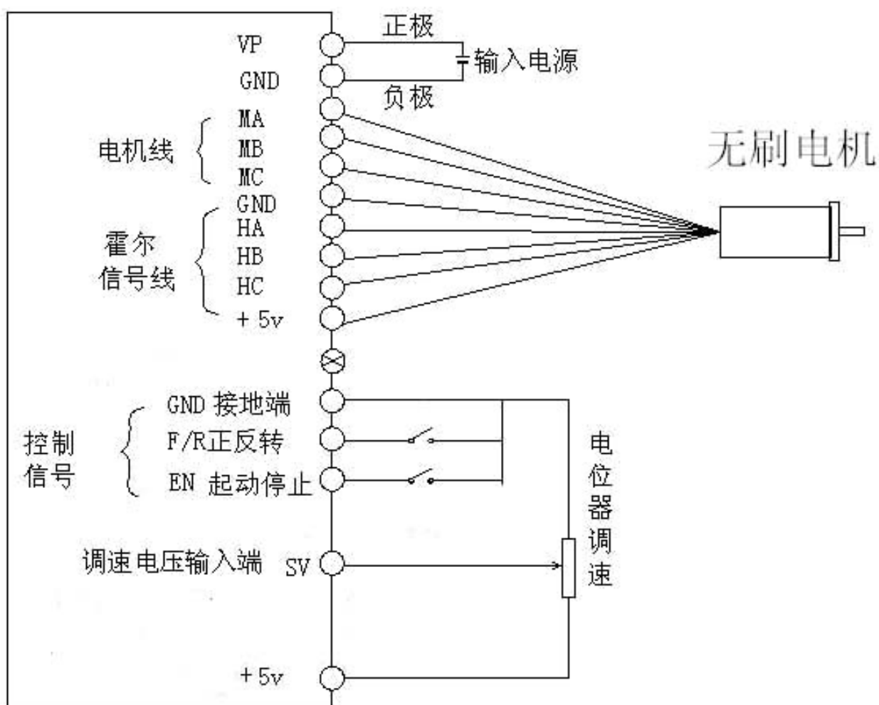
驱动器与无刷电机接线图
